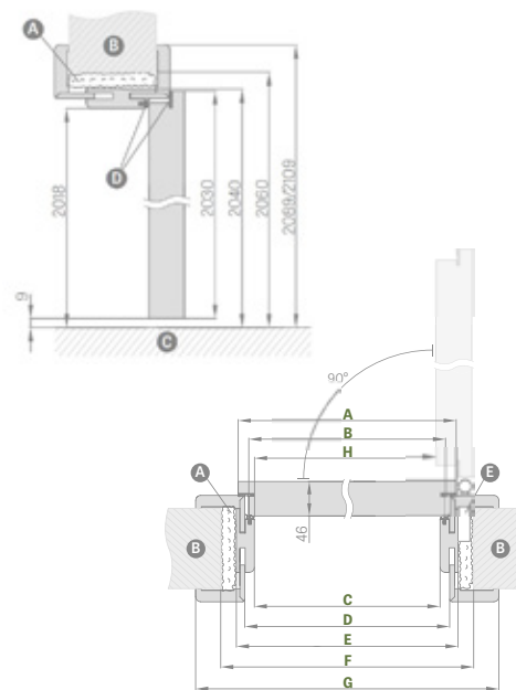
Schéma du dormant réglable
