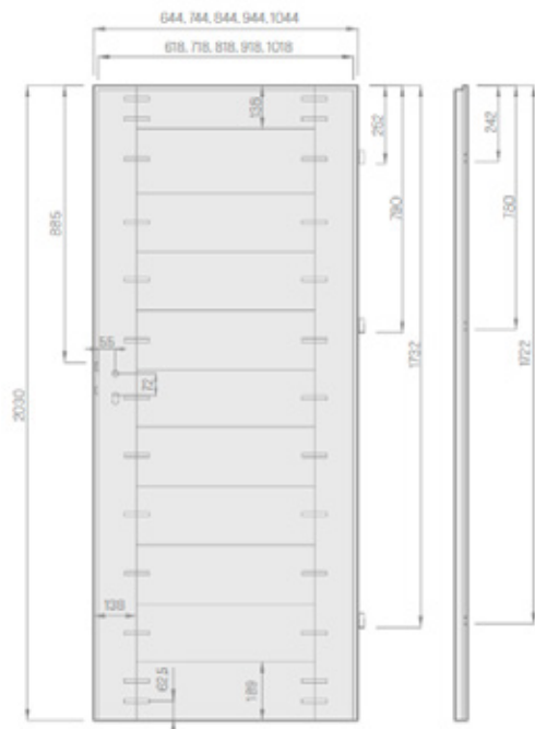
vantail avec les paumelles visibles
