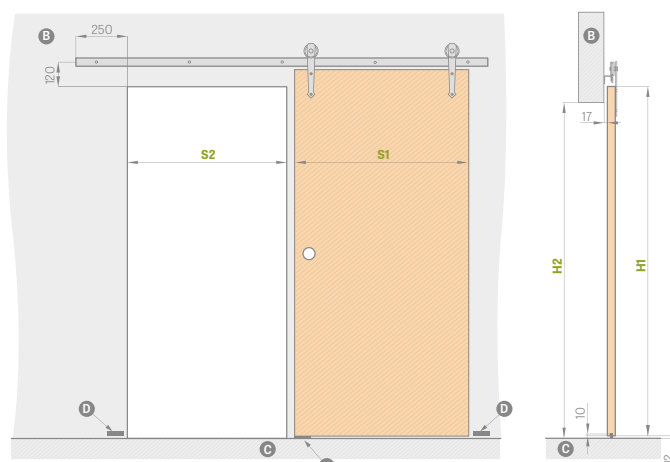
Vantail LOFT, coloris CHÊNE ST CPL, poignée ronde, support pour le vantail RETRO
